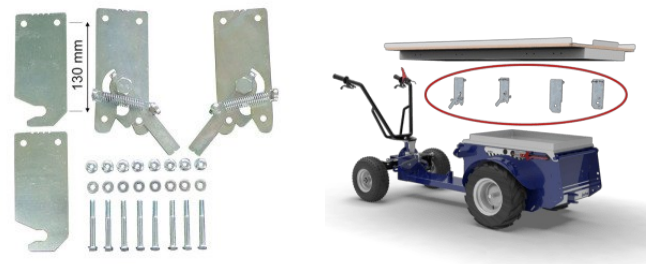
Schnell Befestigungs Kit für Plattform
